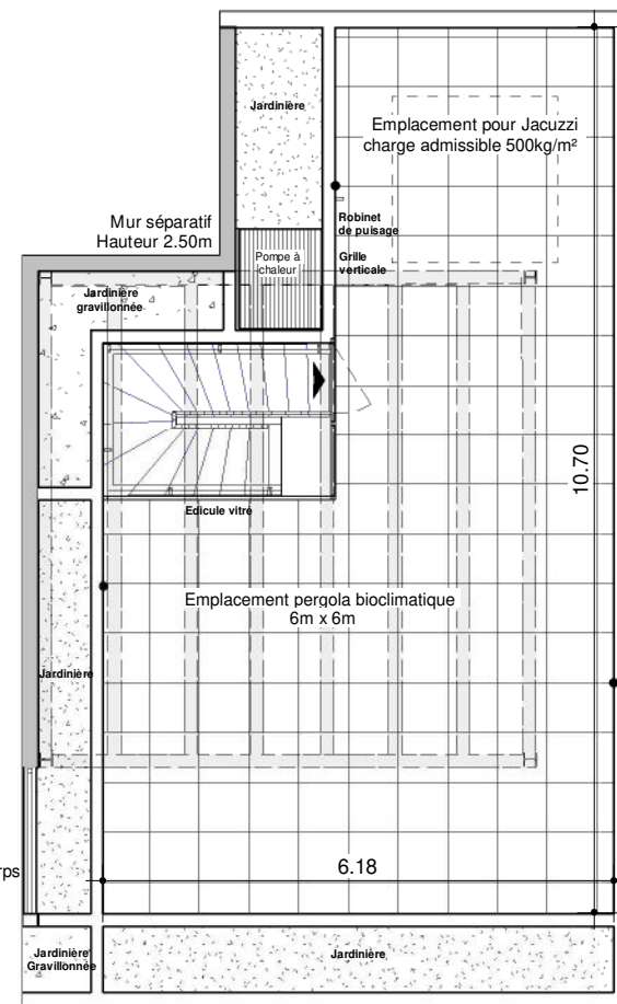
NIVEAU R+9 1/100
