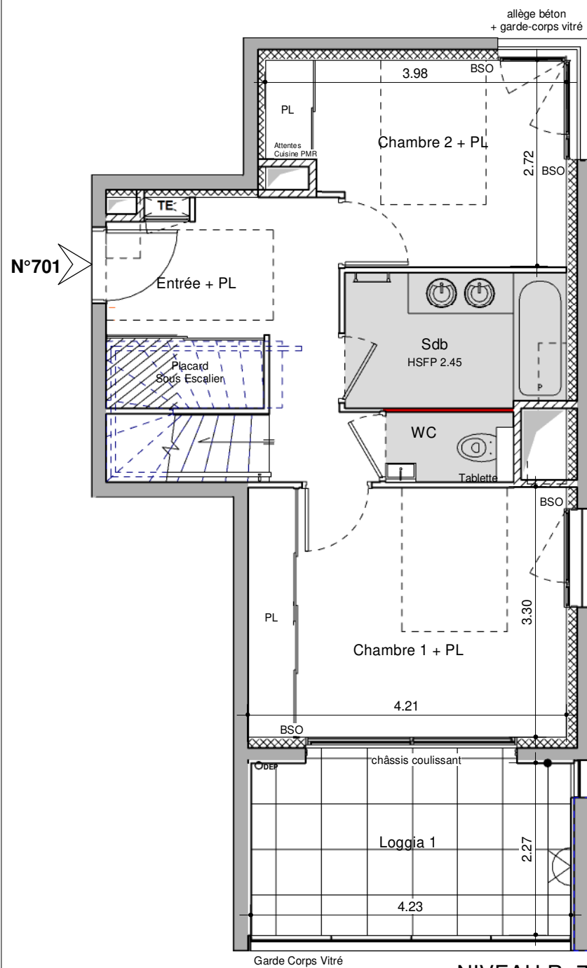
NIVEAU R+7
